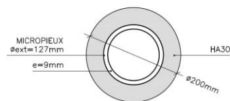
SECTION MICROPIEUX ÉCHELLE 1:5
